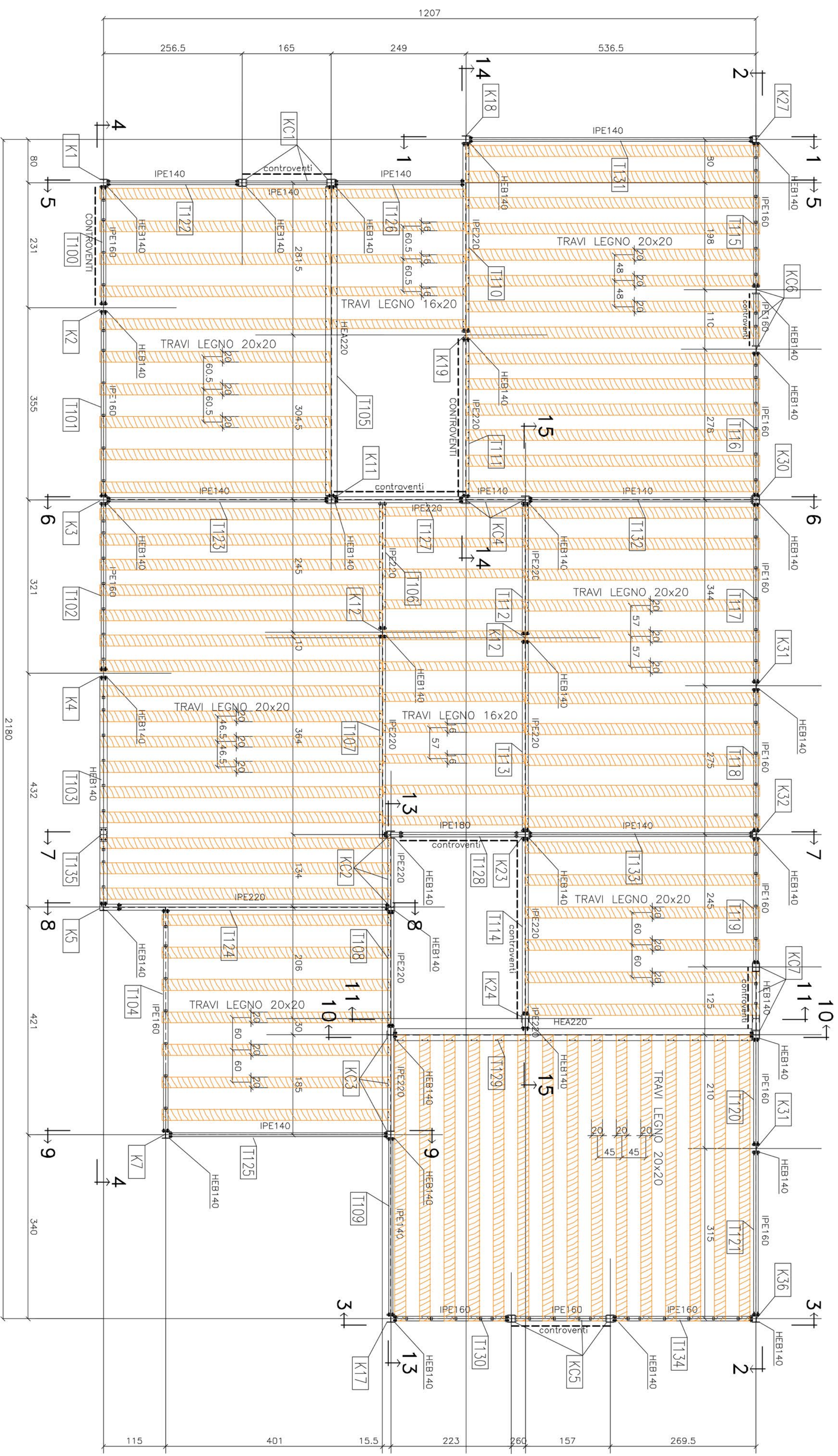
PIANTA 2° SOLAIO
