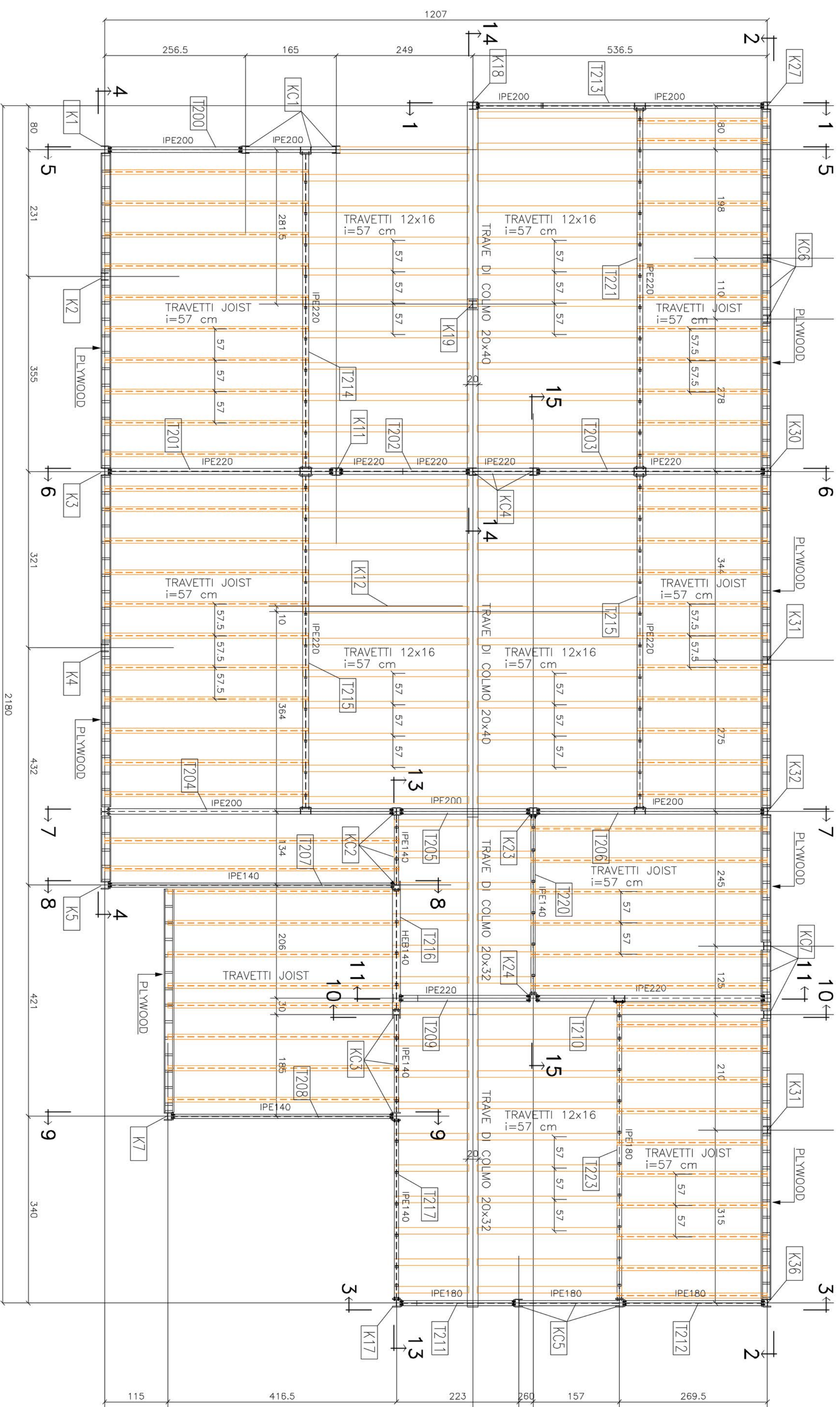
PIANTA COPERTURA
