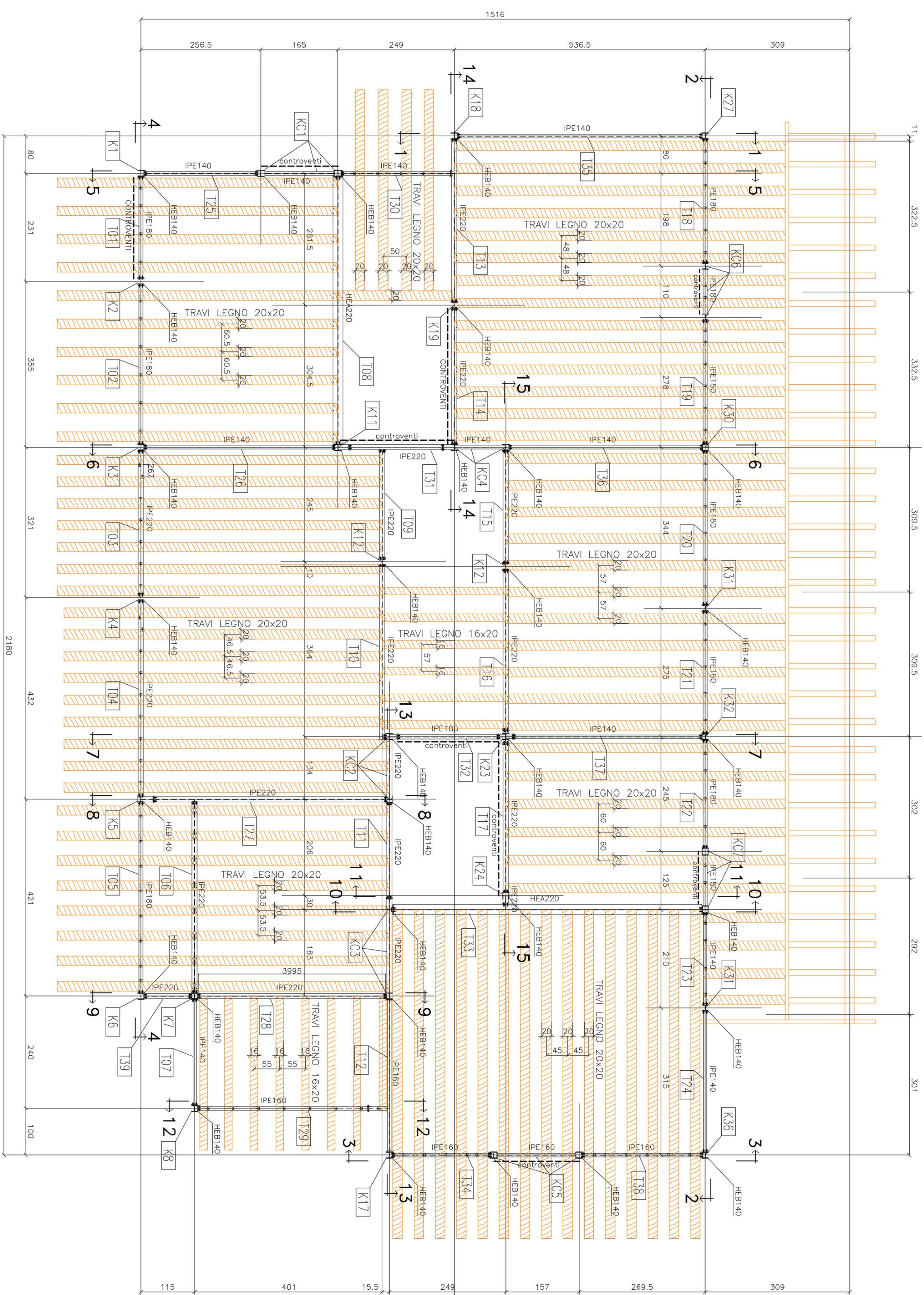
PIANTA 1° SOLAIO
